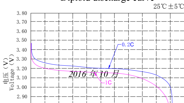
放电曲线图 Diploid discharge curve
